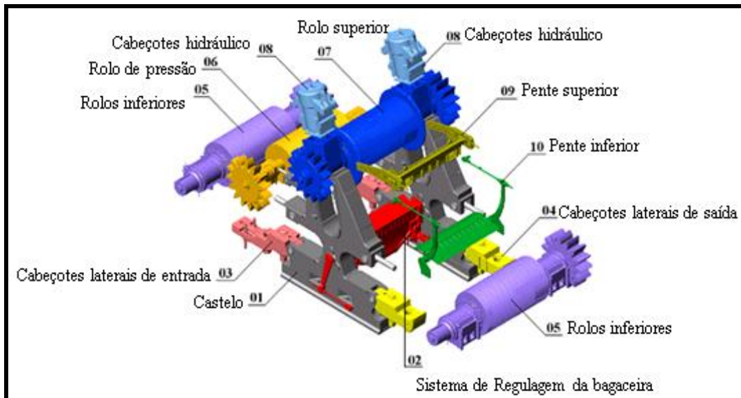
FIGURA 2 – Vista explodida de um terno de moenda
