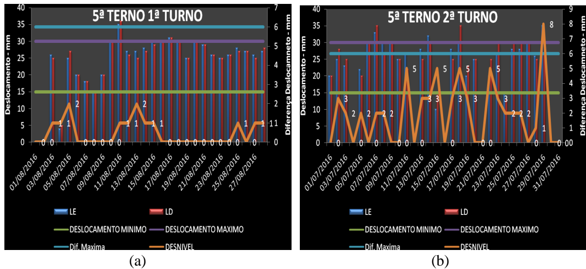
Figura 11 – 5 a terno em operação ideal/Desnivelado
