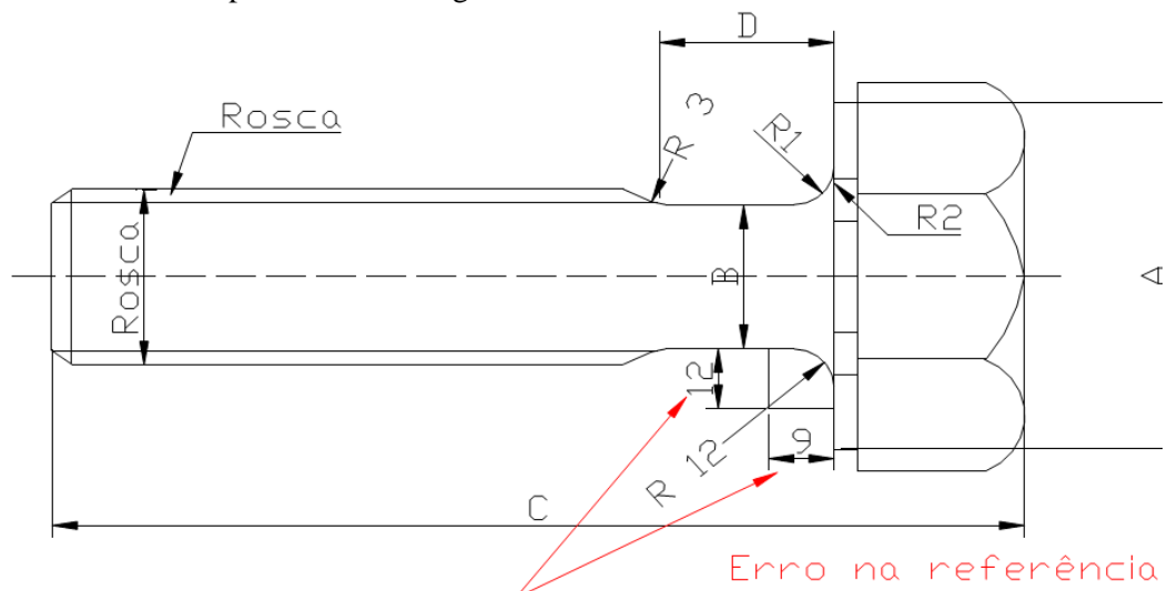
Figura 9 – Geometria dos parafusos do flange da moenda
